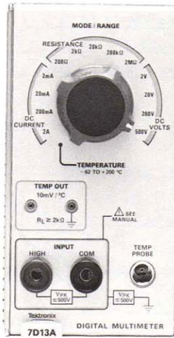
7D13A
