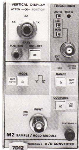
7D12/M2
